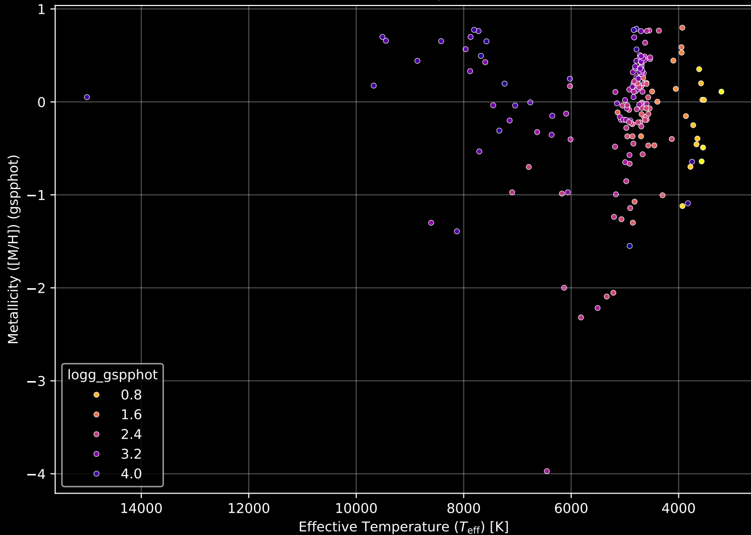
APOGEE DR17 Field: [355-02] Stellar Population Parameters (n= 181)
